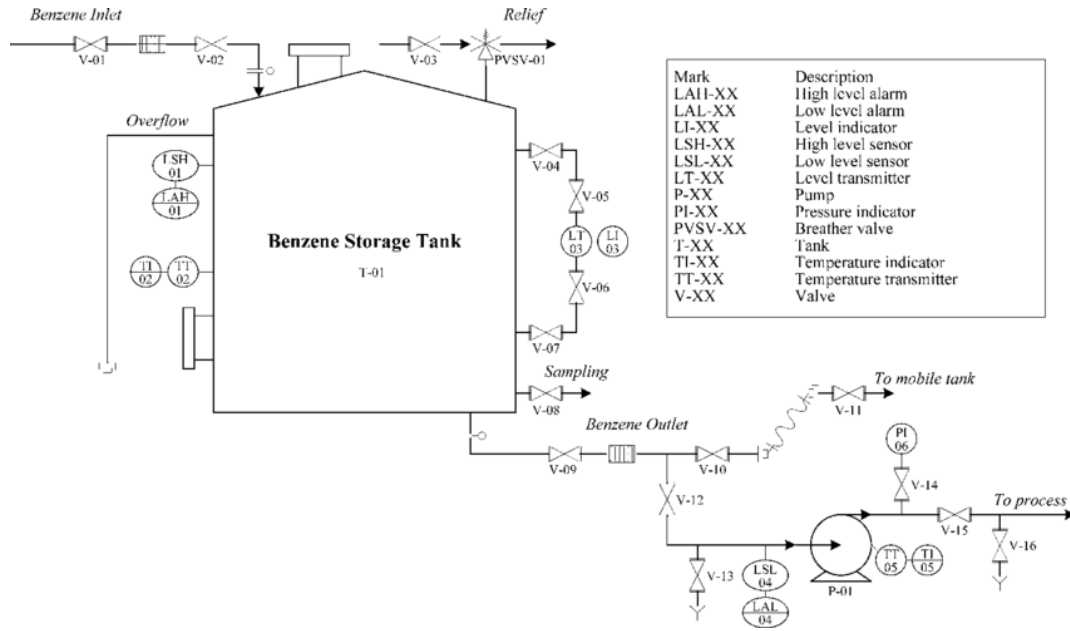
Figure 1.1 : Schéma PID d'un réservoir à toit flottant.
