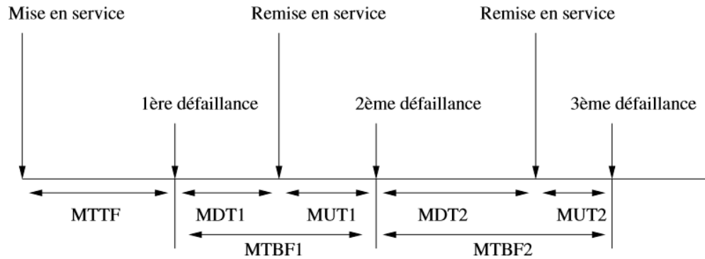
Figure 5.3 : Représentation des temps moyens dans la vie en opération
