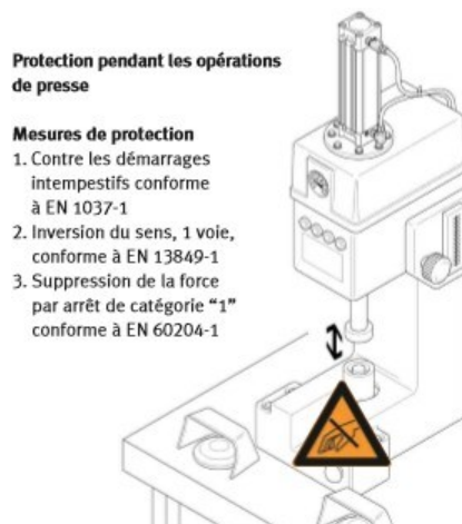
Figure 4.1 : protection pendant les opérations de presse
