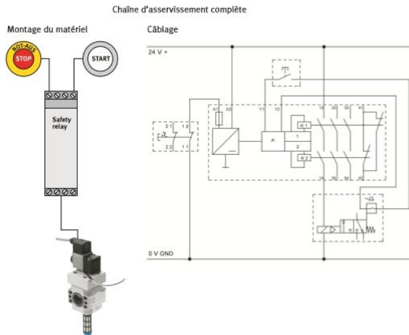
Figure 4.6 : Exemple d'un système d'arrêt d'urgence sur appareil
