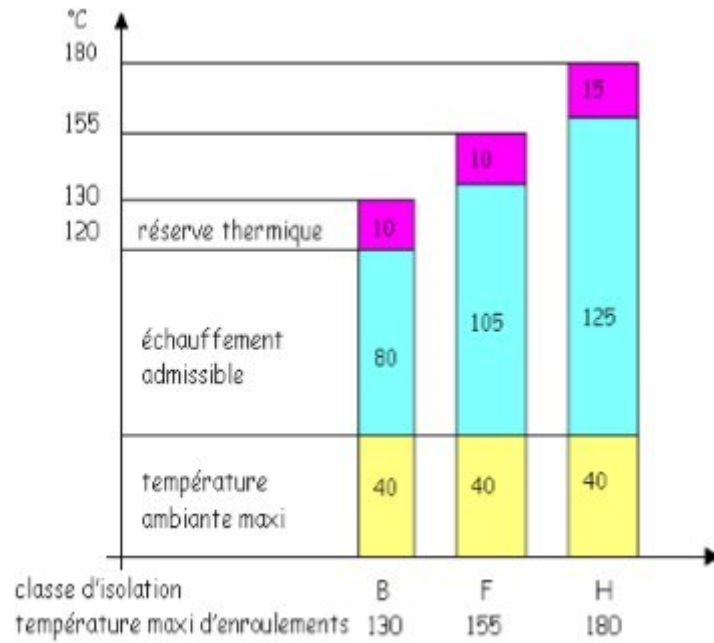
Figure 4.5 : les classes de températures
