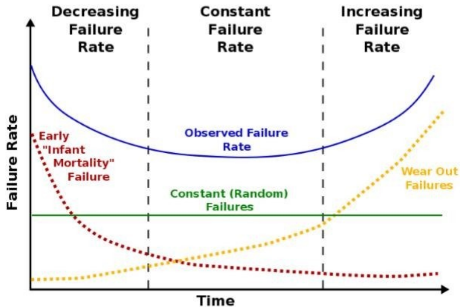
Figure 5.2 : Taux de défaillance en fonction du temps
